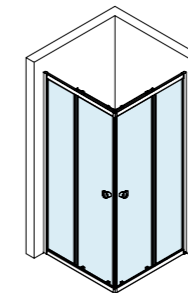
Hoekinstap met schuifdeuren 90x90x200 cm (873-888x873-888 mm)
