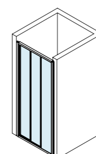
Driedelige schuifdeur 80x200 cm (790-810 mm) 85x200 cm (840-860 mm) 90x200 cm (880-910 mm) 95x200 cm (940-960 mm) 100x200 cm (990-1010 mm)
