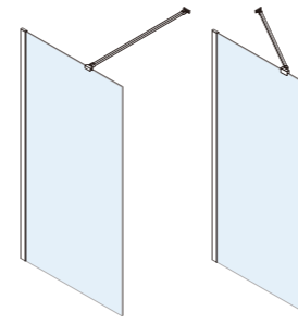
Inloop A3 90 (870-890 mm) 120 (1170-1190 mm)
