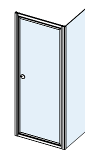
Draai-/schuifdeur met zijwand 80x80 (773-813 x 770-790 mm) 80x90 (773-813 x 870-890 mm) 90x80 (873-913 x 770-790 mm) 90x90 (873-913 x 870-890 mm)
